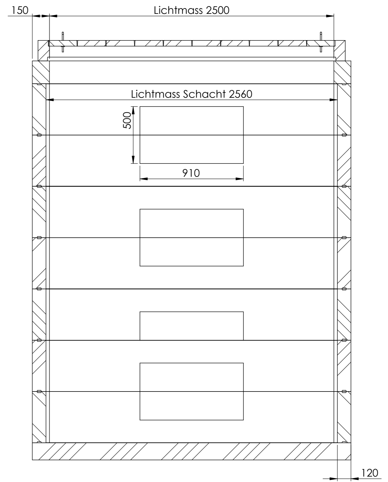
SCHNITT B-B MABSTAB 1 : 20
